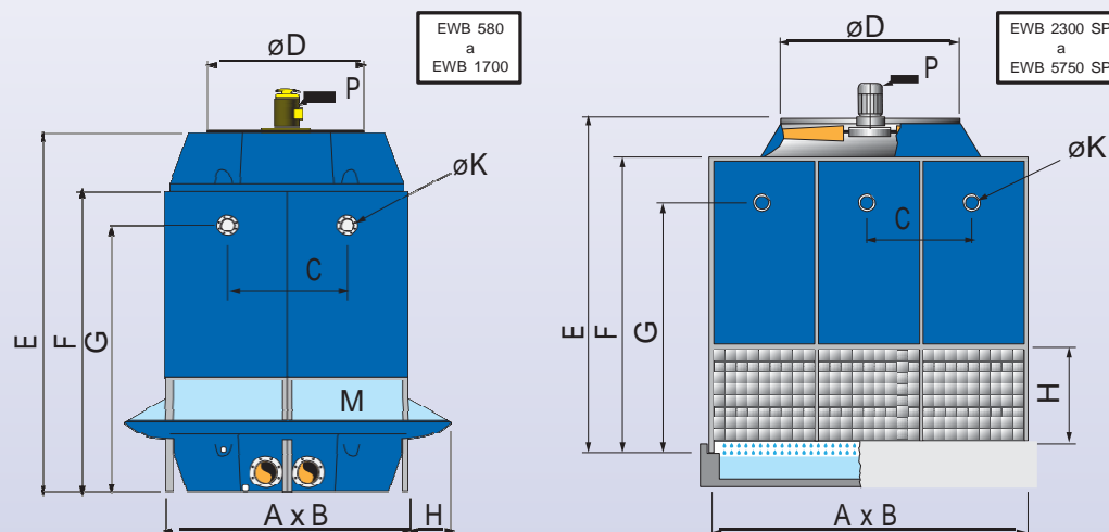
DIMENSIONES DE TORRES TIPO EWB
